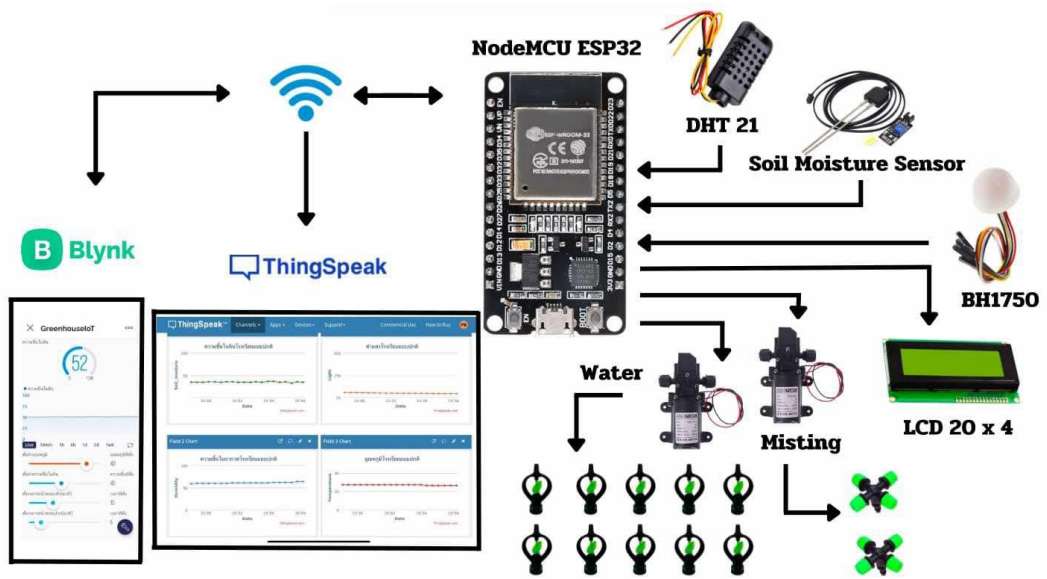
ภาพที่ 2 อุปกรณ์และการเชื่อมต่อในโรงเรือนอัจฉริยะ
