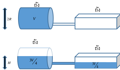
รูปที่ 2 การถ่ายเทของเหลวจากถังทรงกระบอกที่วางตัวในแนวนอนไปยังถังแรงดันด้วยปริมาตร V/4
