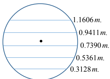
รูปที่ 8 สเกลของระดับของเหลวในถังที่เหลือจากการถ่ายเทของเหลวไปยังถังแรงดันทุกๆ 1.5 ลูกบาศก์เมตร
