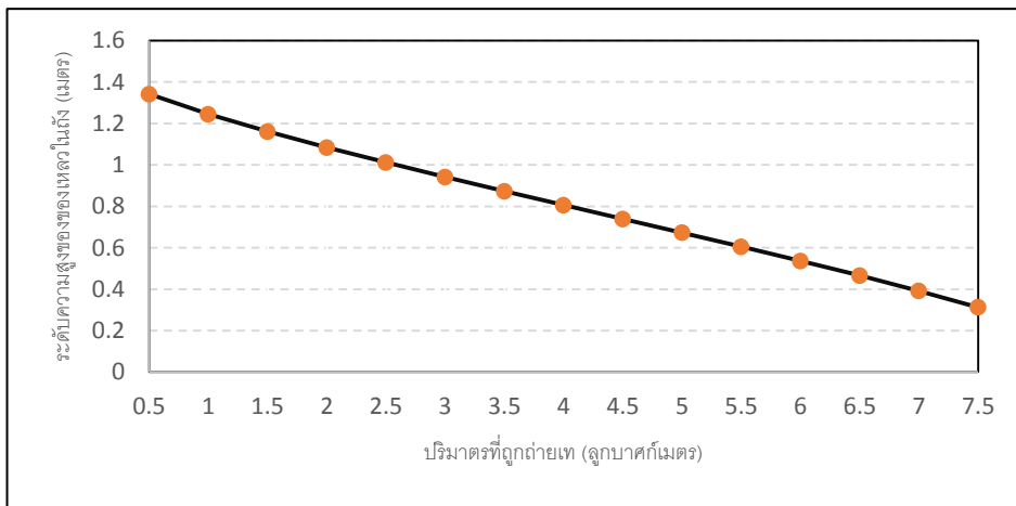
รูปที่ 9 กราฟเส้นคู่อันดับของความสัมพันธ์ระหว่างปริมาตรและระดับความสูงของของเหลวในถัง
