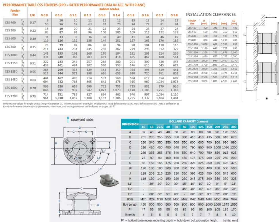
รูปที่ 9 คุณสมบัติของยางกันกระแทก (Fender) และหลักผูกเรือ (Bollard)
