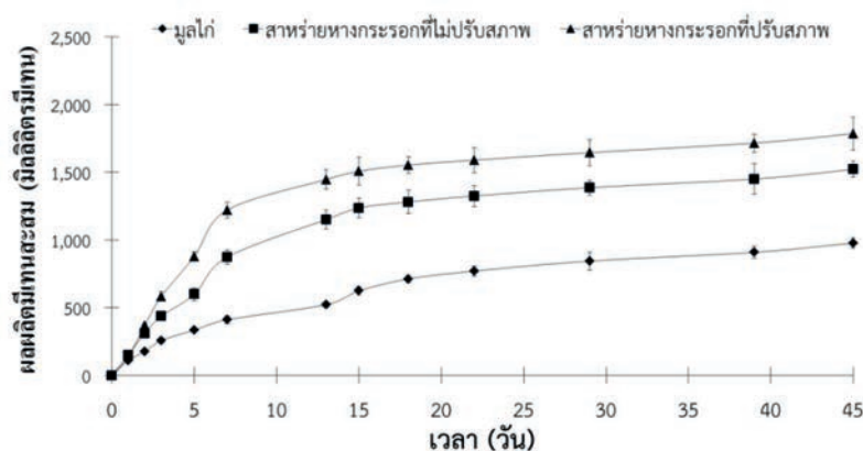
รูปที่ 2 ปริมาณผลผลิตมีเทนสะสมจากการย่อยสลายมูลไก่และสาหร่ายทางกระจกที่ไม่ปรับสภาพและปรับสภาพในสภาวะไร้อากาศ ตั้งแต่ 0-45 วัน
