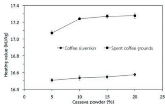
รูปที่ 7 ค่าความร้อนของเชื้อเพลิงอัดเม็ดที่ปริมาณตัว เชื่อมประสานที่แตกต่างกัน
