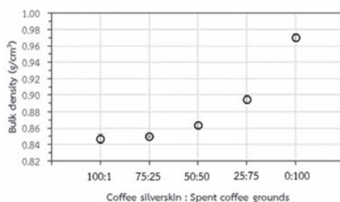
รูปที่ 9 ค่าความหนาแน่นของเชื้อเพลิงอัดเม็ดที่สัดส่วนต่างๆ ของเปลือกหุ้มเมล็ดกาแฟและกากกาแฟ
