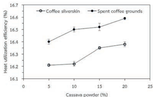
รูปที่ 8 ประสิทธิภาพการใช้งานทางความร้อนของเชื้อเพลิงอัดเม็ดที่ปริมาณตัวเชื่อมประสานที่ต่างกัน
