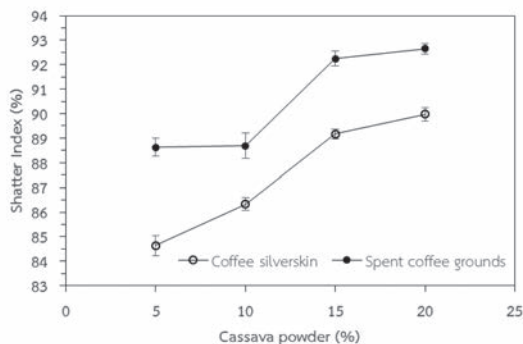
รูปที่ 6 ค่าดัชนีการแตกร่วนของเชื้อเพลิงอัดเม็ดที่ปริมาณตัวเชื่อมประสานที่แตกต่างกัน
