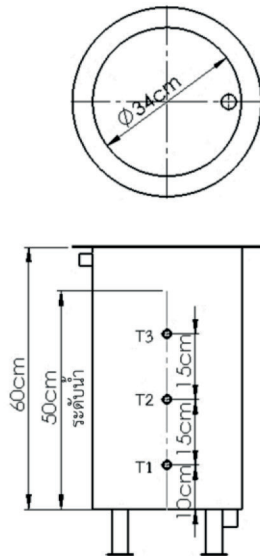
ก) ตำแหน่งวัดอุณหภูมิ
