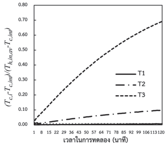
รูปที่ 10 อุณหภูมิของน้ำเมื่อพันท่อน้ำร้อนที่ตำแหน่ง ชิดผนังด้านบน
