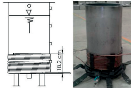
ก) ตำแหน่งซิดผนังด้านล่าง
