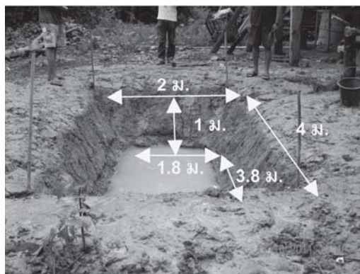
รูปที่ 3 แสดงการจัดเตรียมพื้นที่สำหรับวางถุงหมัก แก๊สชีวภาพ
