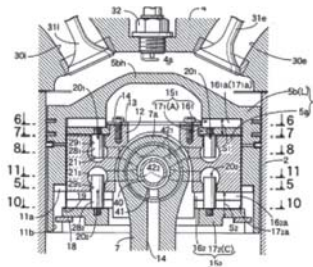
รูปที่ 6 การสร้างลูกสูบสองชั้น
