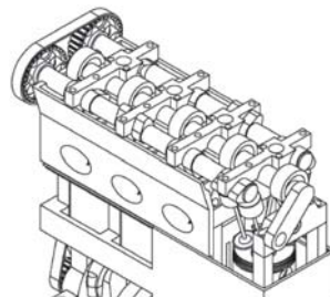
รูปที่ 16 การยกฟาส์ปและเลื้อสับจากด้านบน
