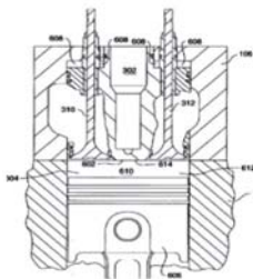
รูปที่ 5 การสร้างห้องเผาไหม้เคลื่อนที่
