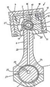
รูปที่ 7 ทางเดินของน้ำมันเครื่องจากเพลาช้อเหวี่ยง
