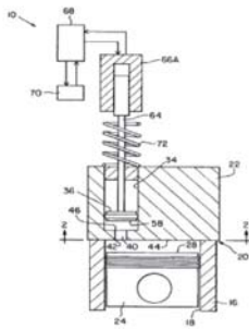
รูปที่ 4 การสร้างห้องเผาไหม้ขนาดเล็ก
