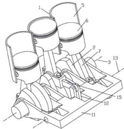
รูปที่ 13 การยกเพลาช้อเหวี่ยงด้วยลูกเบี้ยว
