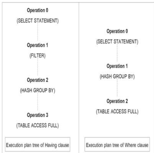
รูปที่ 7 ต้นไม้แสดงขั้นตอนการประมวลผลคำสั่ง เอสคิวแอลโดยใช้ having และ where
