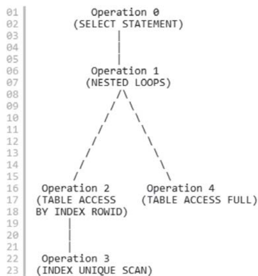
รูปที่ 3 แสดง Execution Plan ในลักษณะของ Tree (Ramsundaram, 2009)
