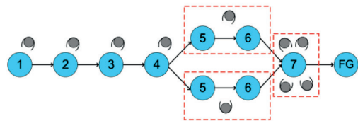
รูปที่ 7 สายการผลิตหลังปรับปรุง (แนวทางที่ 2)
