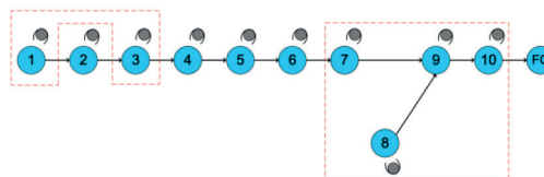
รูปที่ 3 แนวทางการรวมสถานีงาน
