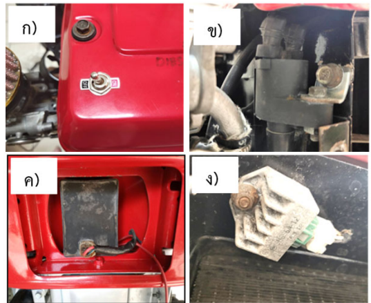
รูปที่ 4 ก) สวิตซ์จุดระเบิด ข) คอยล์จุดระเบิด ค) วงจรควบคุมการจุดระเบิด ง) อุปกรณ์เรียงกระแสไฟ
