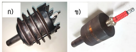
รูปที่ 8 ก) ห้องเผาไหม้เสริมที่ติดตั้งครีบริบายความร้อน ข) ห้องเผาไหม้เสริมของการวิจัยในปี พ.ศ. 2562
