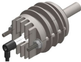
รูปที่ 7 ห้องเผาไหม้เสริมทรงกระบอกที่มีครีบริบายความร้อน
