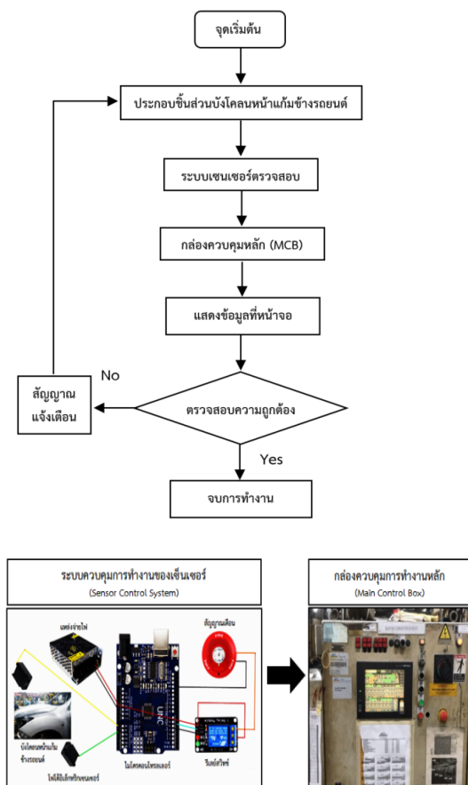
รูปที่ 11 ไดอะแกรมการทำงานของเซ็นเซอร์เพื่อส่งข้อมูลให้กับกล่องควบคุมการทำงานหลัก
