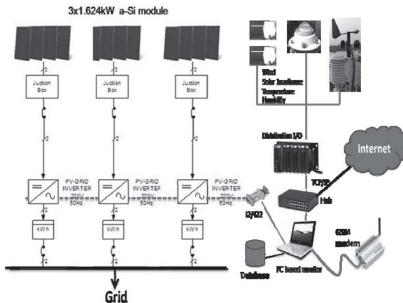
รูปที่ 3 ไดอะแกรมการเชื่อมโยง GSM Modem ร่วมกับระบบเดิม
