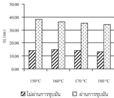
รูปที่ 8 ระยะการยืดตัวที่อุณหภูมิ 150 160 170 และ 180 องศาเซลเซียส เวลา 3 นาที ของผ้าที่ไม่ผ่านการชุบมัน และผ่านการชุบมัน
