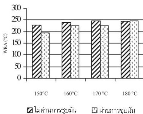
รูปที่ 1 มุมการคืบตัวต่อรอยยับที่อุณหภูมิ 150 160 170 และ 180 องศาเซลเซียส เวลา 2 นาที ของผ้าที่ไม่ผ่านการชุบมัน และผ่านการชุบมัน
