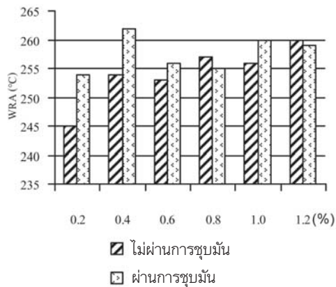
รูปที่ 10 มุมการคืนตัวต่อรอยยับที่ปริมาณความเข้มข้นของโคโคซาน 0.2 0.4 0.6 0.8 1.0 และ 1.2 เปอร์เซ็นต์ อุณหภูมิ 180 องศาเซลเซียส เวลา 3 นาที ของผ้าที่ไม่ผ่านการชุบมันและผ่านการชุบมัน
