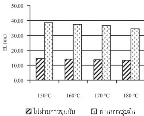
รูปที่ 7 ระยะการยืดตัวที่อุณหภูมิ 150 160 170 และ 180 องศาเซลเซียส เวลา 2 นาที ของผ้าที่ไม่ผ่านการชุบมัน และผ่านการชุบมัน
