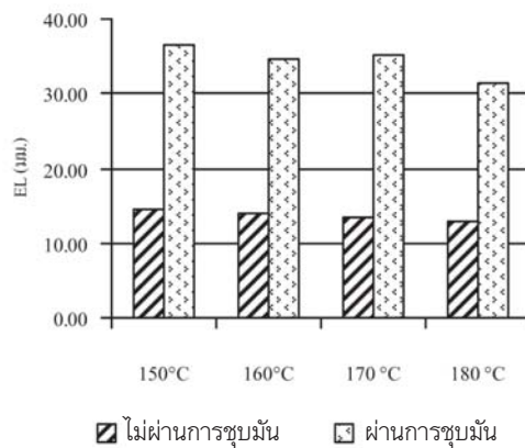
รูปที่ 9 ระยะการยืดตัวที่อุณหภูมิ 150 160 170 และ 180 องศาเซลเซียส เวลา 4 นาที ของผ้าที่ไม่ผ่านการชุบมัน และผ่านการชุบมัน
