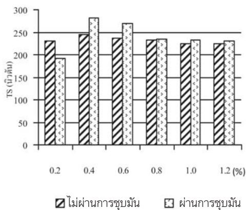
รูปที่ 11 ความทนต่อแรงดึง ที่ปริมาณความเข้มข้นของโคโคซาน 0.2 0.4 0.6 0.8 1.0 และ 1.2 เปอร์เซ็นต์ อุณหภูมิ 180 องศาเซลเซียส เวลา 3 นาที ของผ้าที่ไม่ผ่านการชุบมันและผ่านการชุบมัน
