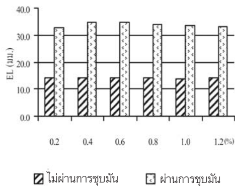
รูปที่ 12 ระยะการยืดตัว ที่ปริมาณความเข้มข้นของโคโคซาน 0.2 0.4 0.6 0.8 1.0 และ 1.2 เปอร์เซ็นต์ อุณหภูมิ 180 องศาเซลเซียส เวลา 3 นาที ของผ้าที่ไม่ผ่านการชุบมันและผ่านการชุบมัน
