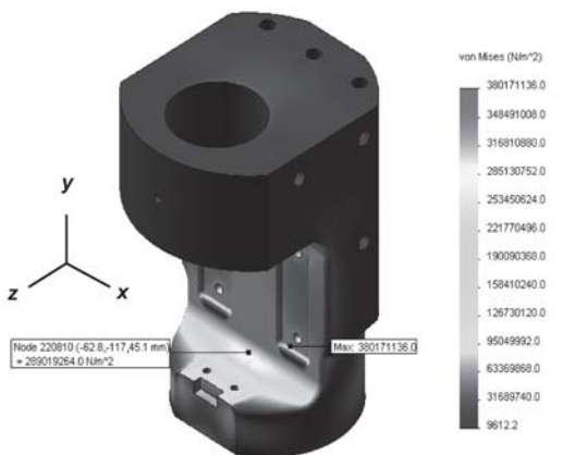
รูปที่ 13 ความเค้นสูงสุดที่ความดัน 300 bar
