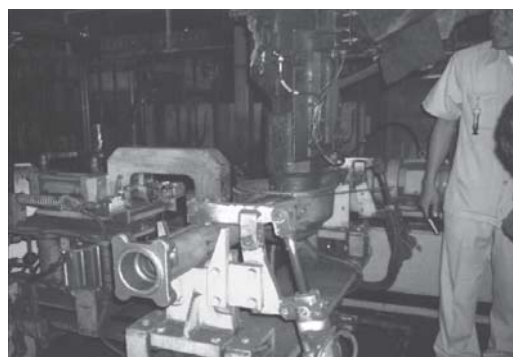
รูปที่ 2 หัวรีฟอร์มกำลังทำการบีบอัดหน้าแปลนเลื้อเพลาลูกหลัง
