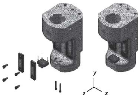
รูปที่ 8 การแบ่งแบบจำลองทางคอมพิวเตอร์ด้วย เอลิเมนต์ Ten nodes tetrahedral
