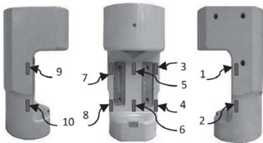
รูปที่ 3 ตำแหน่ง Strain gages ทั้ง 10 ตัว ที่ติดตั้งบนหัวรีฟอร์ม
