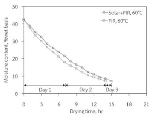
รูปที่ 9 การเปลี่ยนแปลงความชื้นของถ่านอัดแท่งระหว่างการอบแห้งด้วยพลังงานแสงอาทิตย์ร่วมกับรังสีอินฟราเรดไกล และการอบแห้งด้วยรังสีอินฟราเรดไกลเพียงอย่างเดียวที่อุณหภูมิ 60^{\circ}\text{C} โดยอบแห้งในวันที่ 19, 20 และ 21 สิงหาคม 2558 ตั้งแต่เวลา 10.00-17.00 น.
