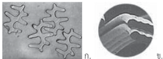
รูปที่ 6 ลักษณะภาคตัดขวางของเส้นใย ก. 4-DG™ (Fiber Innovation Technology, Inc. 2014) และ ข. Waveron® (Teijin Frontier Co., Ltd., 2015)
