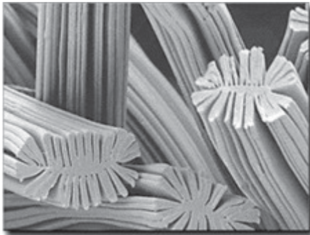
รูปที่ 18 เส้นใยสององค์ประกอบที่ควบคุมรูปร่างของแกนกลางให้เหมาะสมกับการใช้งานด้านการกรองและการดูดซับ (Janet Bealer Rodie, 2012)
