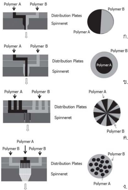
รูปที่ 10 ลักษณะอย่างง่ายของชุดประกอบแผ่นอัดรีดเส้นใย และเส้นใยสององค์ประกอบที่ผลิตได้ ก.ชนิดติดกัน, ข.มีแกนกลาง, ค.เสี้ยว, ง.กระจายตัวในเส้นใย
