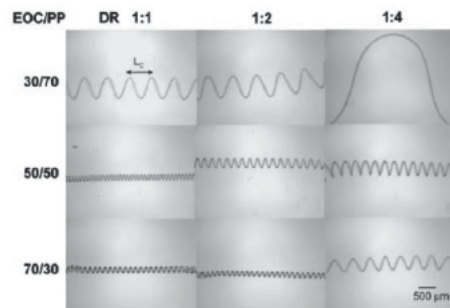
รูปที่ 13 เส้นใยที่เกิดการหยิกงอด้วยตัวเอง จากเส้นใยสององค์ประกอบระหว่าง EOC กับ PP (Chureerat Phahsarn, Wattana Klinsukhon, Nanjaporn Rongpaisan and Natee Srisawat, 2013)
