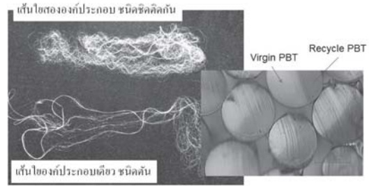
รูปที่ 12 เส้นใยสององค์ประกอบพอลิบูทิลีนเทเรฟทาเลต ชนิดรีไซเคิล (Valox IQ315) (สีเข้ม) กับ ชนิดบริสุทธิ์ (Valox 315) (สีอ่อน) ชนิดติดกัน (นที ศรีสวัสดิ์, 2556)
