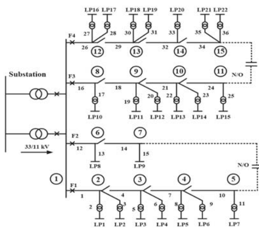
รูปที่ 2 ระบบจำหน่ายไฟฟ้าทดสอบ RTBS บัส 2
