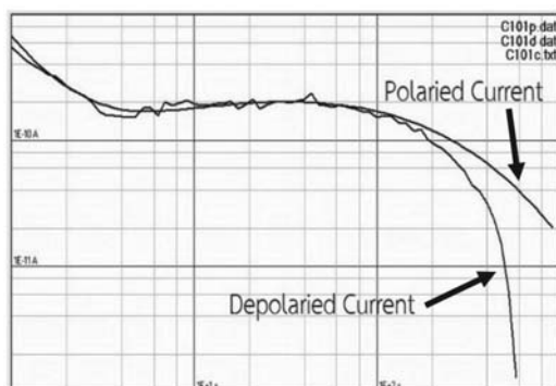
รูปที่ 6 ผลการทดสอบบุชชิงด้วย PDC
