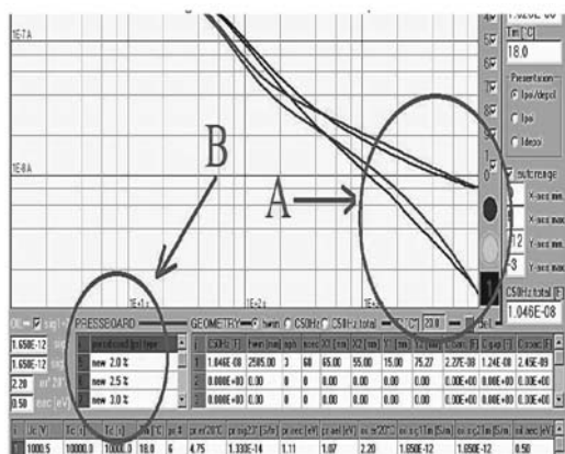
รูปที่ 11 ส่วนปลายของกราฟกระแสโพลาร์ไรซ์และ ดีโพลาร์ไรซ์เป็นตัวบ่งชี้ค่าความชื้นของอุปกรณ์ ที่ทดสอบ
