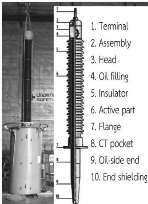
รูปที่ 8 ตัวอย่างขูซึ่งหม้อแปลงไฟฟ้าแรงสูง
