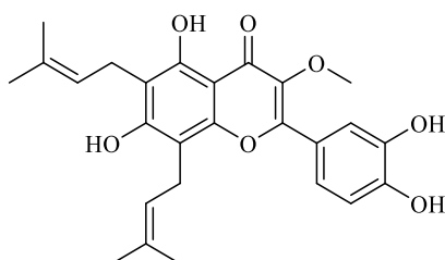
2-(3,4-Dihydroxy-phenyl)-5,7-dihydroxy-3-methoxy-8-((E)-3-methyl-but-2-enyl)-6-(3-methyl-but-2-enyl)-1-benzopyran-4-one
