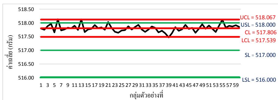
รูปที่ 1 น้ำหนักในกระบวนการบรรจุเปรียบเทียบกับข้อกำหนดน้ำหนักของครีมอาบน้ำฟอกขนนกแก้ว
