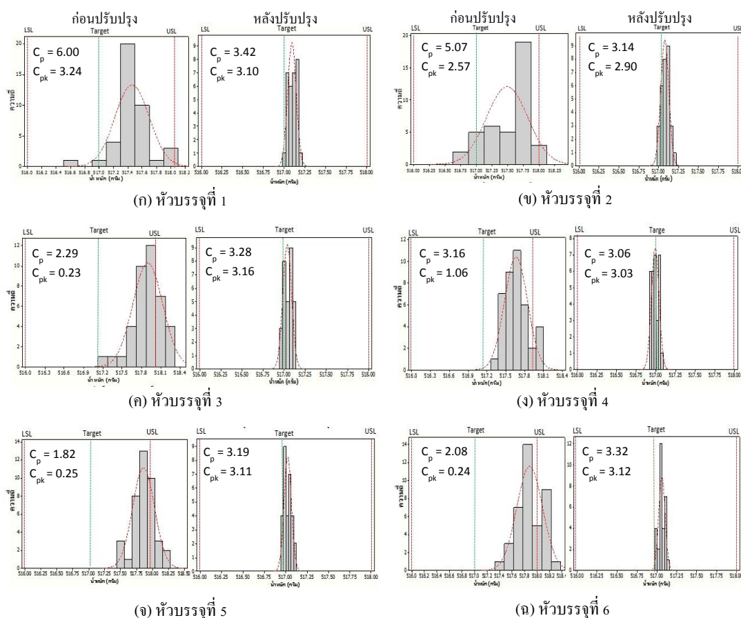
รูปที่ 10 ค่าเฉลี่ยของกระบวนการผลิตครีมน้ำพุดกาน นกแก้วจากหัวบรรจุ 6 หัว ก่อนและหลังปรับปรุง
