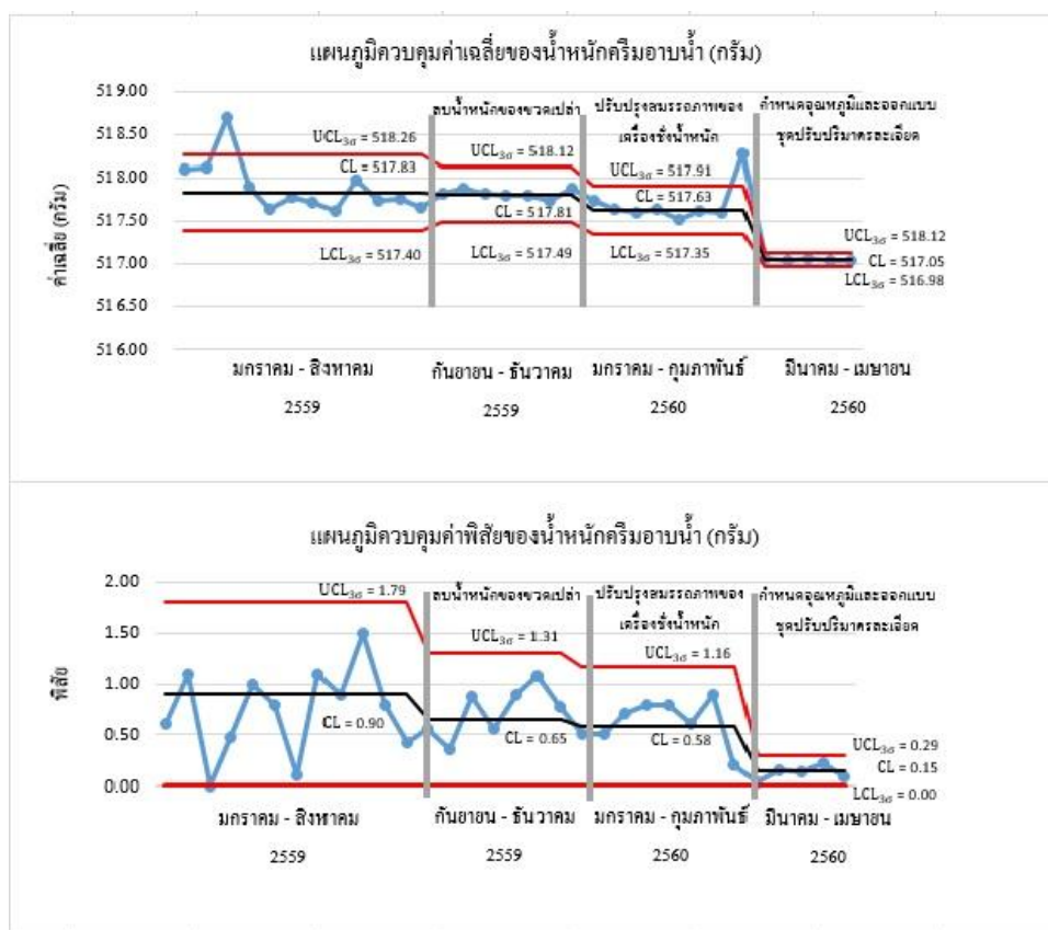
รูปที่ 11 ความแตกต่างของค่าเฉลี่ยและพิสัยในกระบวนการบรรจุครีมอาบน้ำก่อนและหลังการปรับปรุง
