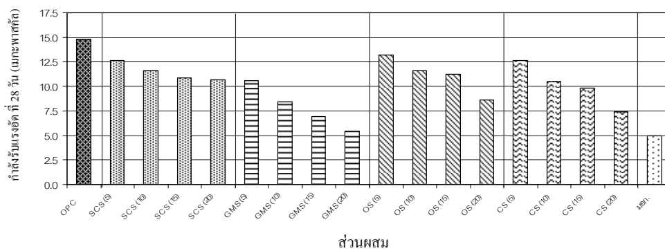
รูปที่ 11 กําลังอัดของมอร์ตาร์ผสมเปลือกหอยบด
