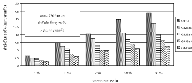
รูปที่ 10 กำลังอัดของมอร์ตาร์ผสมเปลือกหอยแมลงภู่นบด
