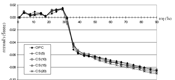
รูปที่ 15 การหดตัวแบบแห้งของมอร์ตาร์ผสมเปลือกหอยแครงบด
