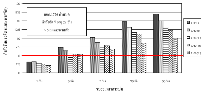
รูปที่ 8 กำลังอัดของมอร์ตาร์ผสมเปลือกหอยนางรมบด
