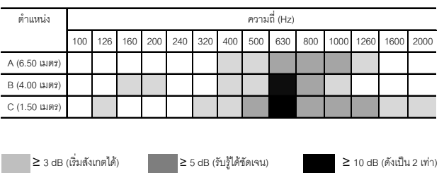
รูปที่ 22 ความแตกต่างของระดับเสียงที่วัดได้ ก่อนและหลังติดตั้งวัสดุดูดกลืนเสียง ตามการทดลองกรณี S2
