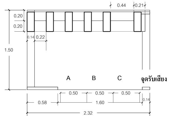
รูปที่ 4 แบบจำลองบริเวณใต้คานของสถานีรถไฟฟ้าบีทีเอส
