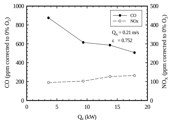
รูปที่ 7 อิทธิพลของอัตราการจ่ายเชื้อเพลิงที่มีต่อ CO และ NO_x ที่สภาวะ \varepsilon = 0.752 และ Q_A = 0.21 m/s
