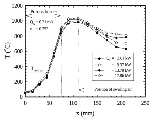
รูปที่ 6 โครงสร้างทางอุณหภูมิตามแนวแกนของหัวพ่นไฟ ที่สภาวะ \varepsilon = 0.752 และ Q_A = 0.21 m/s
