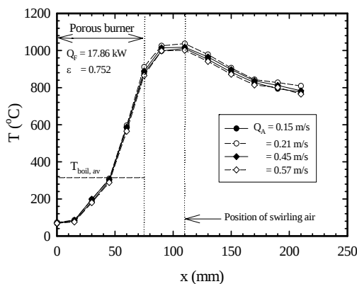
รูปที่ 4 โครงสร้างทางอุณหภูมิตามแนวแกนของหัวพ่นไฟ ที่สภาวะ \varepsilon = 0.752 และ Q_F = 17.86 kW
