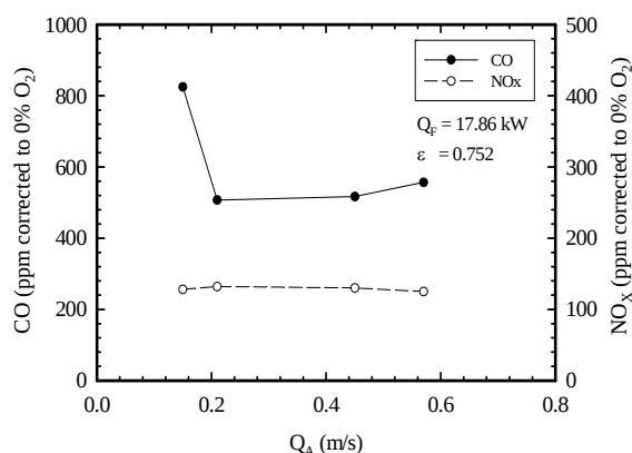
รูปที่ 5 อิทธิพลของอัตราการจ่ายอากาศหมุนวนที่มีต่อ CO และ NO_x ที่สภาวะ \varepsilon = 0.752 และ Q_F = 17.86 kW
