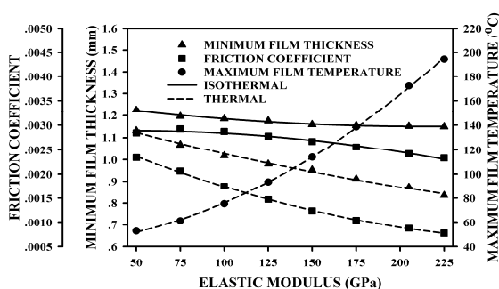
รูปที่ 15 ความหนาฟิล์มน้อยสุด สัมประสิทธิ์ความเสียดทาน และอุณหภูมิของฟิล์มสารหล่อลื่นสูงสุดเมื่อทรงกระบอกมีค่าอีลาสติคโมดูลัสต่างๆ
