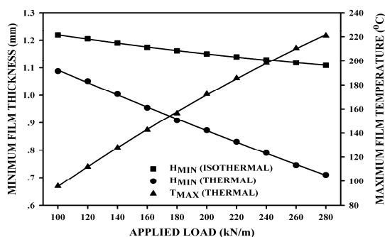
รูปที่ 8 ความหนาฟิล์มน้อยสุดและอุณหภูมิสูงสุดของฟิล์มสารหล่อลื่นเมื่อทรงกระบอกรับภาระต่างๆ
