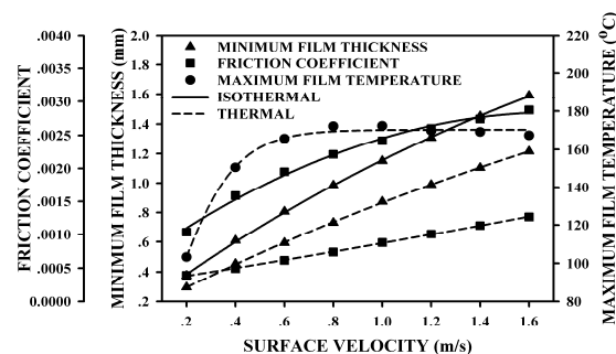
รูปที่ 12 ความหนาฟิล์มน้อยสุด อุณหภูมิสูงสุดของฟิล์มสารหล่อลื่นและสัมประสิทธิ์ความเสียดทาน เมื่อความเร็วของทรงกระบอกต่างๆ
