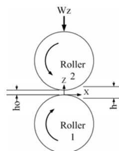
รูปที่ 1 ลักษณะของทรงกระบอกและฟัดที่ใช้ในการจำลองผล
