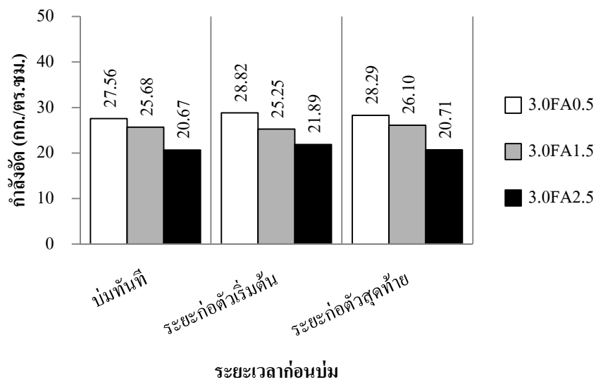
รูปที่ 5 กำลังอัดของอีโพอキシเรซินที่อัดตัวจากบ่มเตาอบไฟฟ้า 80 °C
