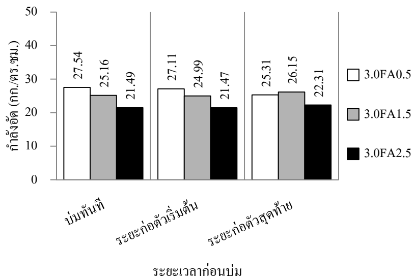
รูปที่ 4 กำลังอัดของอีโพอキシเรซินที่อัดตัวจากบ่มเตาอบไฟฟ้า 60 °C
