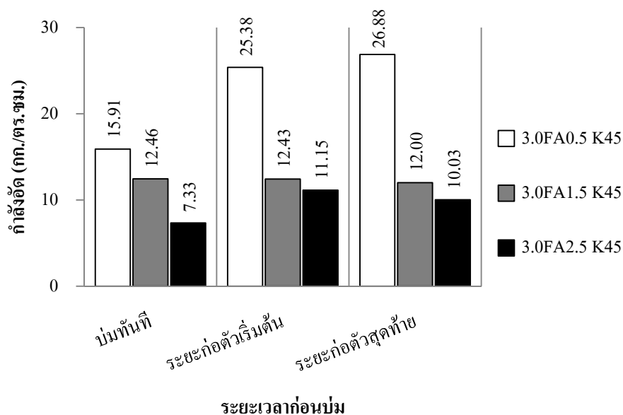
รูปที่ 7 กำลังอัดของจีโอโพลิเมอร์มอร์ตาร์จากการบ่มเตอบไมโครเวฟ 60 °C คงอุณหภูมิ 45 นาที
