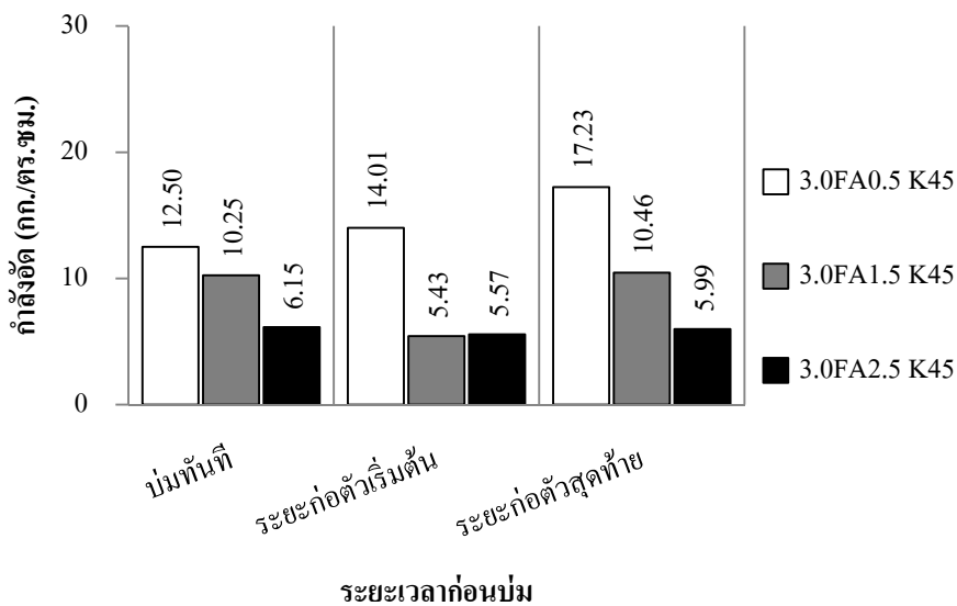
รูปที่ 6 กำลังอัดของจีโอโพลิเมอร์มอร์ตาร์จากการบ่มเตอบไมโครเวฟ 40 °C คงอุณหภูมิ 45 นาที
