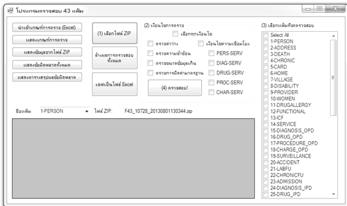
รูปที่ 6 หน้าจอหลักโปรแกรมตรวจสอบคุณภาพข้อมูล 43 แฟ้ม
