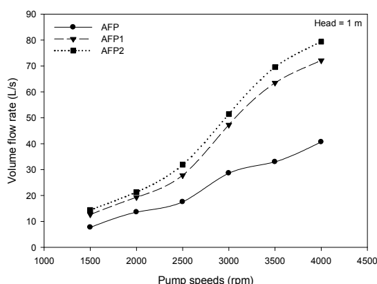
รูปที่ 6 ความสัมพันธ์ระหว่างอัตราการไหลและความเร็วรอบของ AFP, AFP1 และ AFP2 ที่เฮด 1 เมตร
