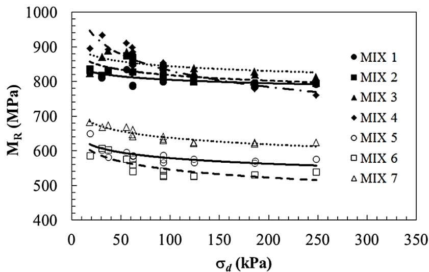
รูปที่ 6 ผลการทดสอบค่าโมดูลัสคืบตัว ( M_R )
