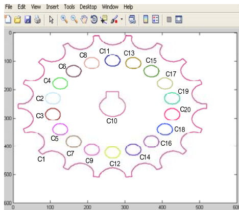
รูปที่ 7 เส้นโครงร่างของเฟืองล้อจักรยาน
