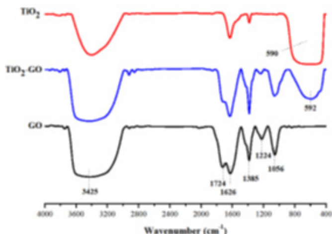
Figure 5 The FT-IR spectra of GO, TiO 2 -GO and TiO 2 composites.
