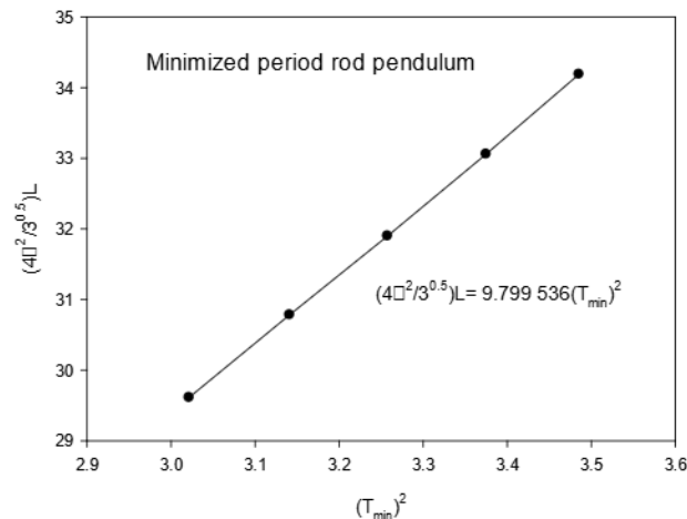
รูปที่ 9 ความสัมพันธ์ระหว่าง (4\pi^2/3^{0.5})L กับ T_{\min}^2 ของลูกตุ้มแท่งกลมที่มีคานน้อยที่สุด
