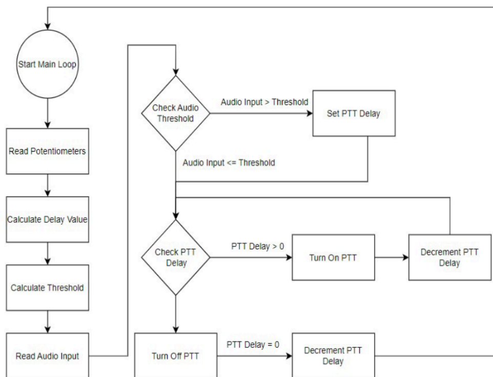
รูปที่ 3 ไอคะแกรมหลักการทำงานของเรดิโอโอเวอร์ไอพี
