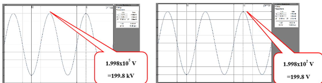
รูปที่ 7 สัญญาณของแรงดันไฟฟ้าคกร้อมตัวเก็บประจุภาคแรงดันสูงและแรงดันไฟฟ้าคกร้อมภาคแรงดันต่ำ
