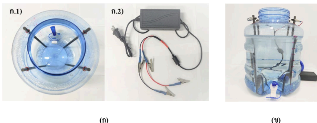
รูปที่ 3 (ก) ชุดอุปกรณ์ผลิต: ก.1) ถังเครื่องผลิตพร้อมแท่งแกรไฟต์ (ขั้วอิเล็กโทรด) และ ก.2) ชุดให้กระแสไฟฟ้า (ข) การใช้งาน: ปฏิริยาไฟฟ้าเคมีที่ขั้วอิเล็กโทรดเกิดก๊าซ H_2(g) , O_2(g) และ Cl_2(g)
