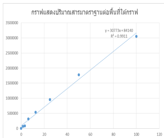
รูปที่ 1 กราฟแสดงความสัมพันธ์ระหว่างความเข้มข้นของสารและพื้นที่ใต้กราฟที่วิเคราะห์โดยเครื่อง HPLC
