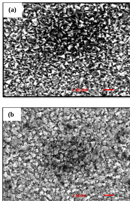
รูปที่ 3 ภาพลักษณะพื้นผิวจากเครื่อง SEM ของขั้วไฟฟ้า (a) Cu 2 O, (b) CuO
