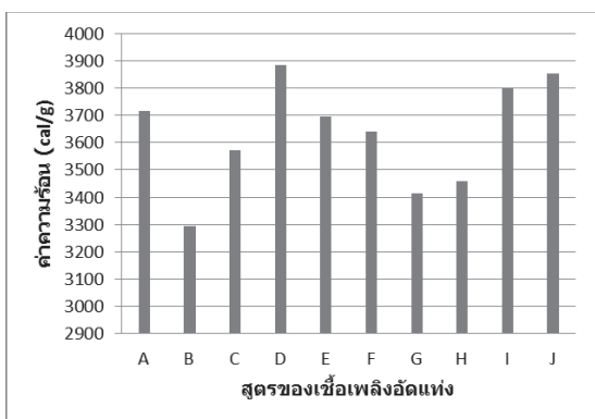
(b) ค่าความร้อนของเชื้อเพลิงอัดแท่ง ภาพที่ 4 สมบัติทางกายภาพของเชื้อเพลิงอัดแท่ง
