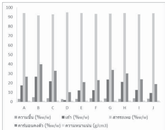
(a) ค่าความชื้น ถ้า สารระเหย คาร์บอนคงตัว และความหนาแน่นของเชื้อเพลิงอัดแท่ง
