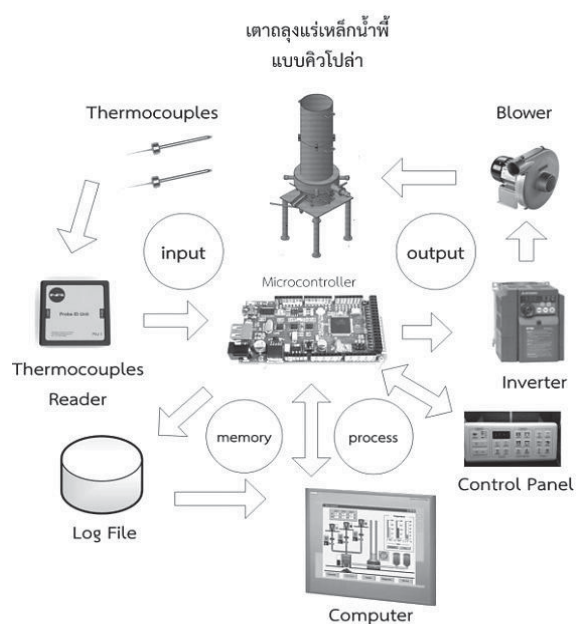
ภาพที่ 1 ภาพรวมของระบบควบคุมอัตโนมัติสำหรับเตาถลุงสินแร่เหล็กน้ำพี้แบบคิวโปลา
