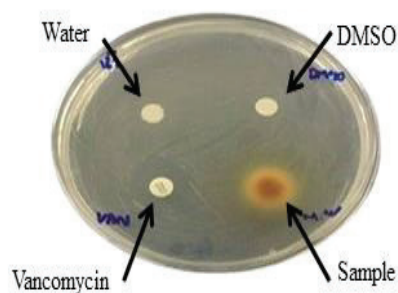
S. typhimurium
