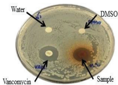
E. coli
