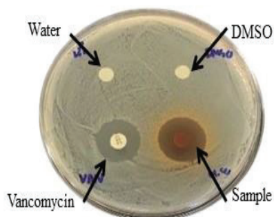
B. cereus
