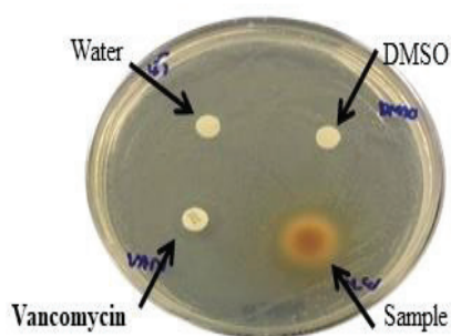
B. subtilis
