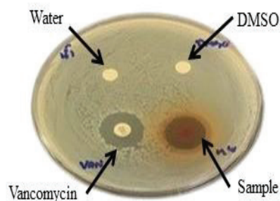
S. aureus
