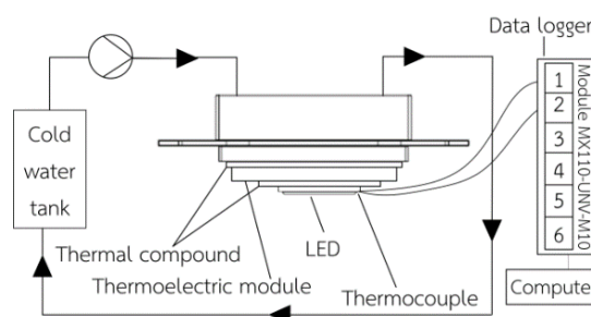
ภาพที่ 3 ไดอะแกรมการทำงานของชุดทดลอง
