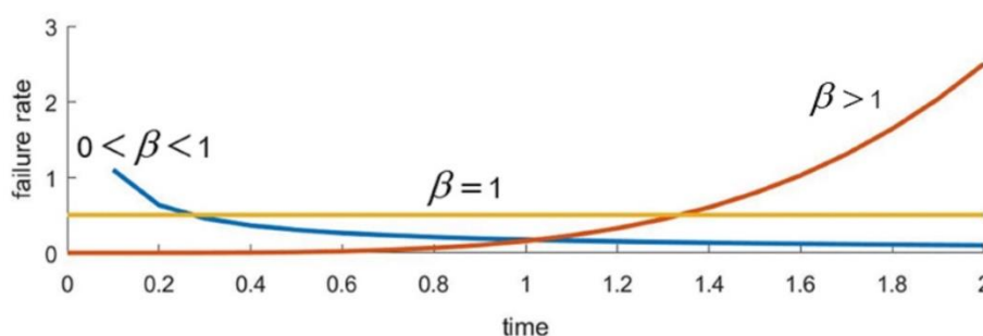
ภาพที่ 2 ความสัมพันธ์ระหว่างพารามิเตอร์รูปร่างของการแจกแจงแบบไวบูลล์กับอัตราการเสีย
