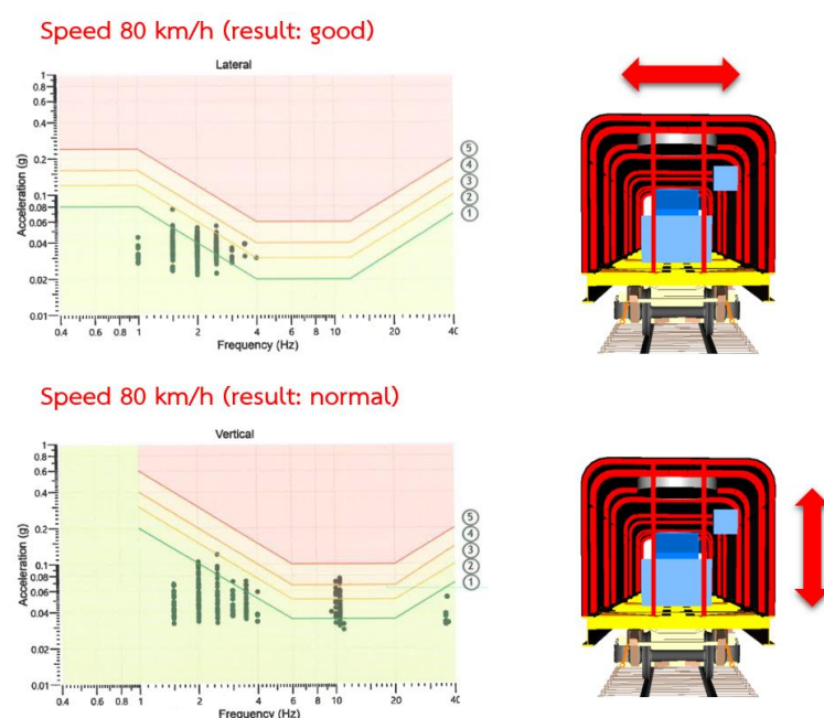
ภาพที่ 7 ผลการประเมินความสะดวกสบายของการโดยสาร (Riding Comfort Test) ตามมาตรฐานของการรถไฟฯ
