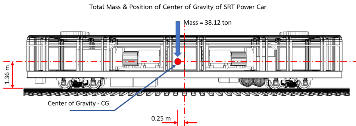
ภาพที่ 4 การวิเคราะห์ตำแหน่งของจุดศูนย์ถ่วงของรถไฟฟ้ากำลัง [11]
