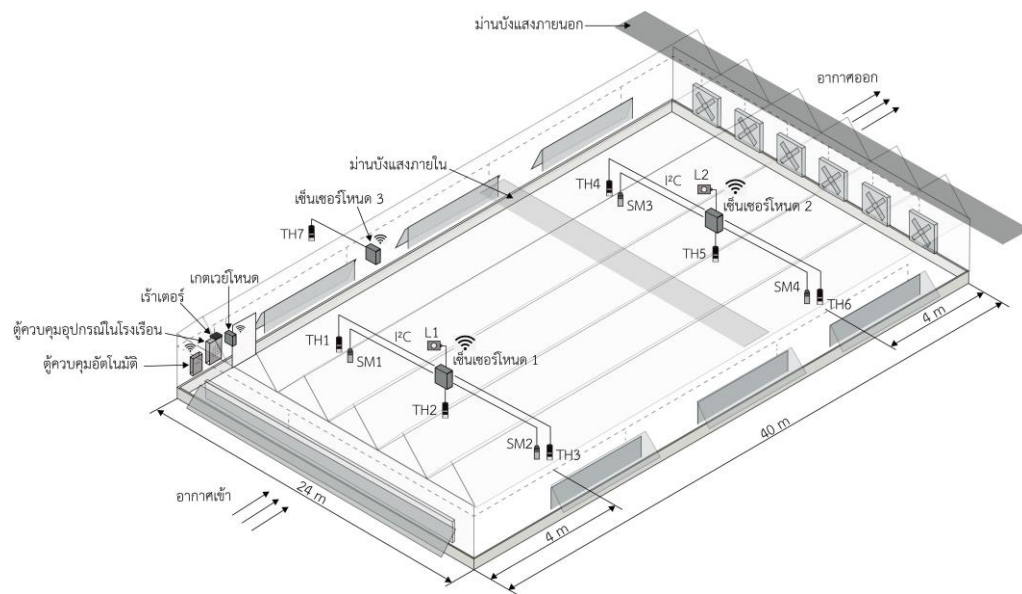
ภาพที่ 3 ตำแหน่งการติดตั้งอุปกรณ์ต่าง ๆ ของระบบควบคุมอัตโนมัติสำหรับโรงเรือนเกษตรอินทรีย์
