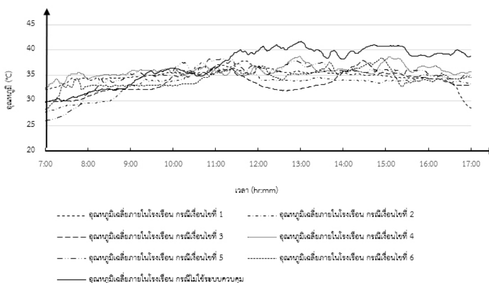
ภาพที่ 11 ผลการทดลองควบคุมอุณหภูมิภายในโรงเรือนของการควบคุมอัตโนมัติแบบมีเงื่อนไข
