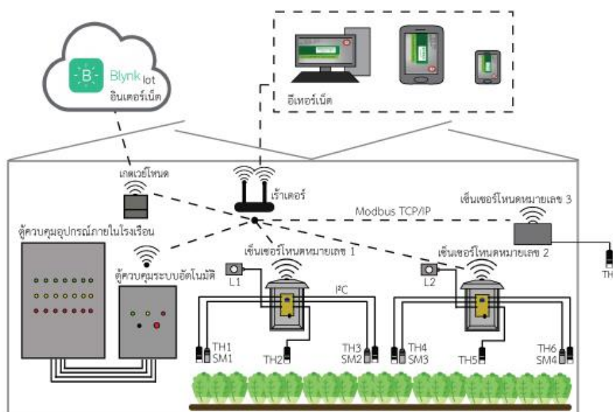
ภาพที่ 2 โดอะแกรมการทำงานของระบบควบคุมอัตโนมัติสำหรับโรงเรือนเกษตรอินทรีย์
