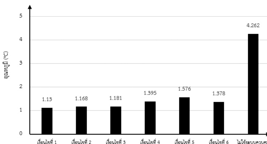
ภาพที่ 12 ค่ารากที่สองของค่าความผิดพลาดกำลังสองเฉลี่ยของอุณหภูมิเฉลี่ยภายในโรงเรือนของทุกเงื่อนไข
