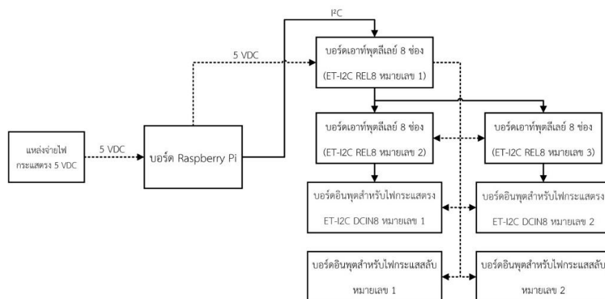
ภาพที่ 4 ไดอะแกรมการทำงานของส่วนต่าง ๆ ภายในตัวควบคุมระบบอัตโนมัติ
