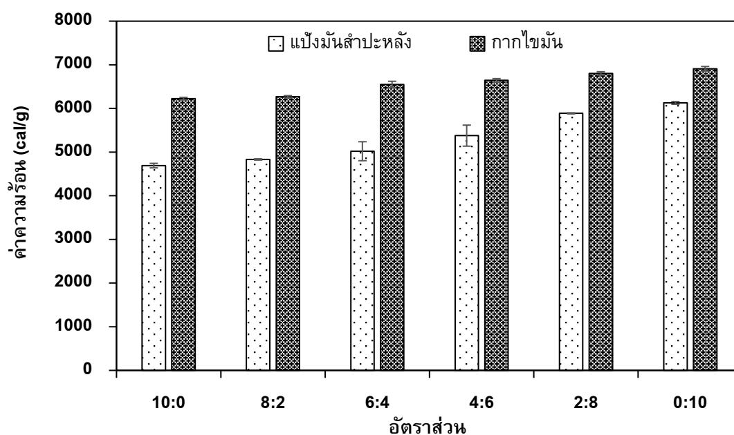
ภาพที่ 4 เปรียบเทียบค่าความร้อนของถ่านอัดแท่งที่ใช้แป้งมันสำปะหลังและกากไขมันเป็นตัวประสาน
