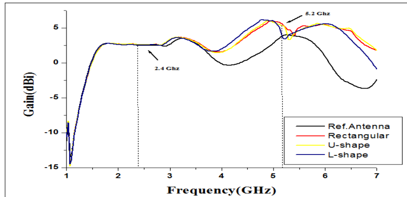
ภาพที่ 19 อัตราขยายของสายอากาศรูปทรงทั้ง 3 แบบ
