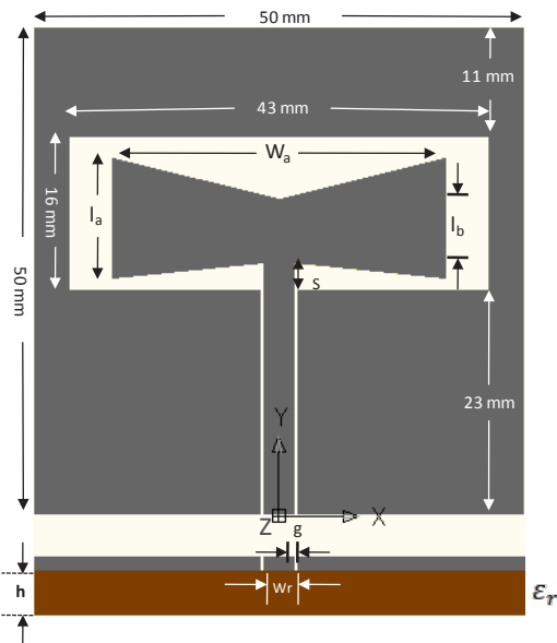
ภาพที่ 1 โครงพื้นฐานในการสร้างสายอากาศ สัตรูปโบ
