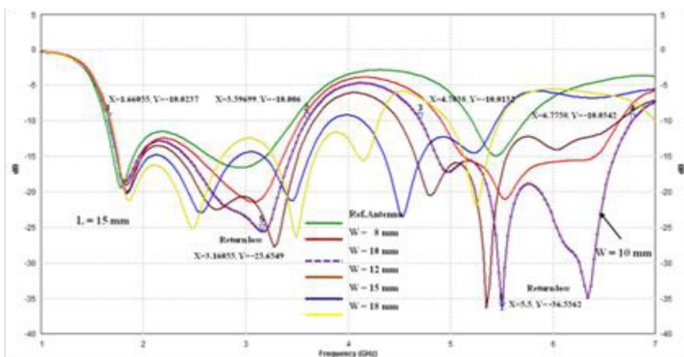
ภาพที่ 5 ค่าสูญเสียย้อนกลับของสายอากาศเมื่อปรับความกว้าง W ของร่องประกอบรูปสี่เหลี่ยม
