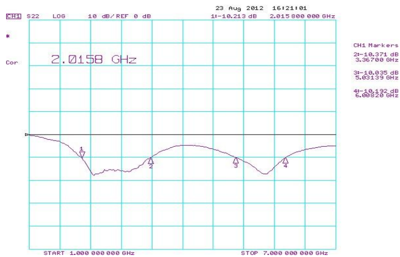
ภาพที่ 15 วัดค่าอิมพีแดนซ์แบนด์วิดท์ของสายอากาศร่องประกรรูปสี่เหลี่ยม [a]
