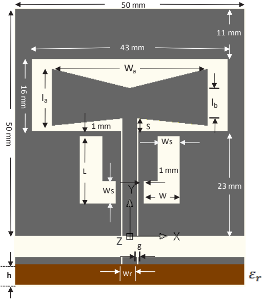
ภาพที่ 4 สายอากาศร่องประกอบรูปตัวแอล
