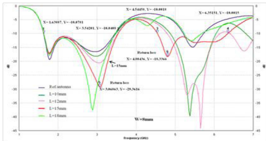
ภาพที่ 12 ค่าสูญเสียย้อนกลับของสายอากาศเมื่อปรับความยาว L ของร่องประกบรูตัวแอล
