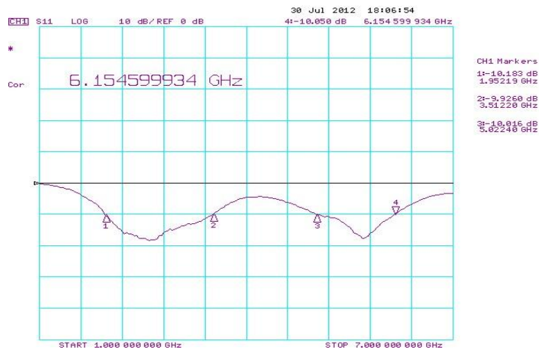
ภาพที่ 16 วัดค่าอิมพีแดนซ์แบนด์วิดท์ของสายอากาศร่องประกรรูปตัวยู [b]
