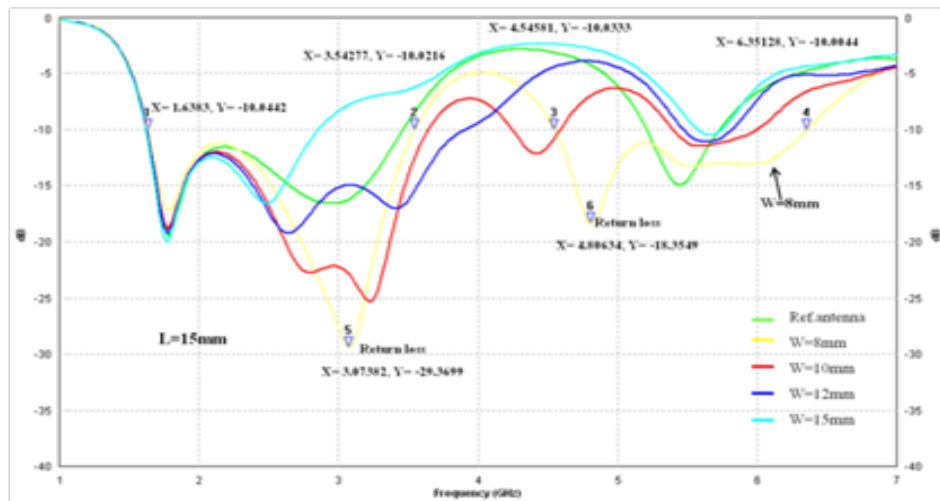
ภาพที่ 11 ค่าสูญเสียย้อนกลับของสายอากาศเมื่อปรับความกว้าง W ของร่องประกบรูตัวแอล
