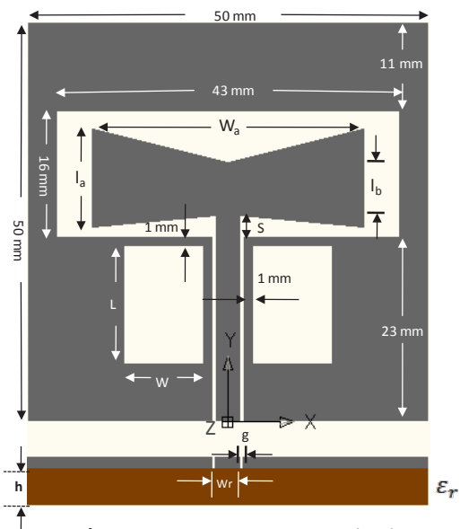
ภาพที่ 2 สายอากาศร่องประกอบรูปสี่เหลี่ยม
