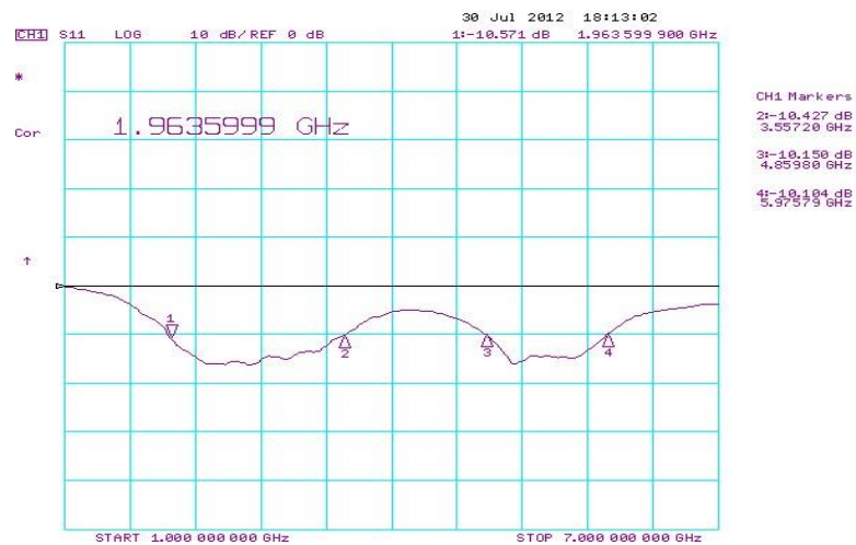
ภาพที่ 17 วัดค่าอิมพีแดนซ์แบนด์วิดท์ของสายอากาศร่องประกรรูปตัวแอล [c]
