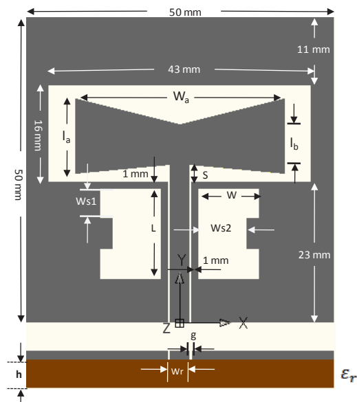
ภาพที่ 3 สายอากาศร่องประกอบรูปตัวยู
