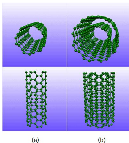
ภาพที่ 1 แบบจำลองโครงสร้าง (a) ท่อนาโนคาร์บอนแบบผนังชั้นเดียวและ (b) ท่อนาโนคาร์บอนแบบผนังหลายชั้น
