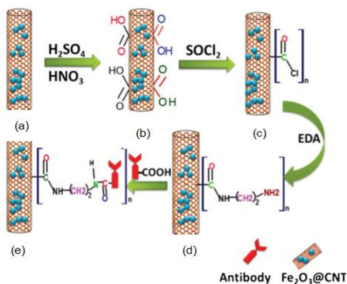
ภาพที่ 3 แสดงกลไกการเติมแอนติบอดี (Antibody) บน Fe_2O_3@CNTs (a) สังเคราะห์ Fe_2O_3@CNT (b) เติมหมู่ -COOH บน Fe_2O_3@CNT (c) SOCl_2 ถูกเติมบน Fe_2O_3@CNT (d) -NH_2 ถูกเติมบน Fe_2O_3@CNT (e) เติมแอนติบอดี (Antibody) [7]
