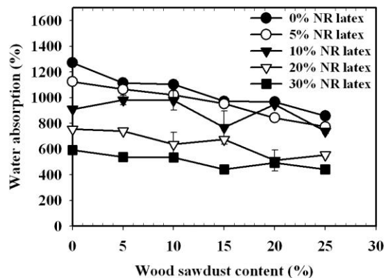
ภาพที่ 6 ความสัมพันธ์ระหว่างค่าการดูดซับน้ำของคอมพอสิตโฟมแข็งกับปริมาณผงซีลี้อยไม้ยางพารา และปริมาณน้ำยางพารา ที่ 25 องศาเซลเซียสนาน 150 นาที
