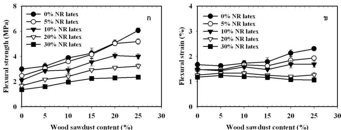
ภาพที่ 5 สมบัติการรับแรงดัดของคอมพอสิตโฟมแบ่งกับปริมาณผงซีลี้อยไม้ยางพารา และปริมาณน้ำยางพารา ก) ค่าการทนต่อแรงดัดสูงสุด และ ข) ค่าการยืดตัว ณ แรงดัดสูงสุด
