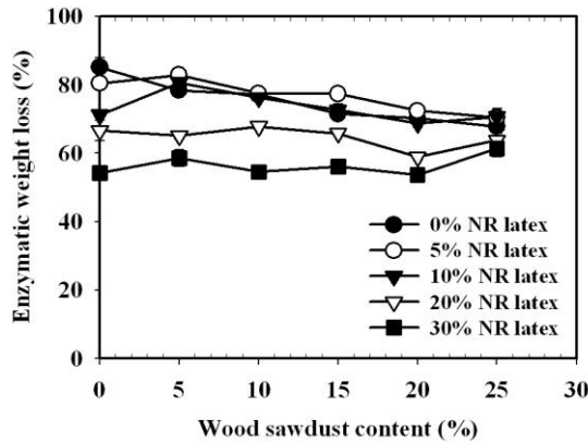
ภาพที่ 7 ความสัมพันธ์ระหว่างค่าการสลายตัวเนื่องจากเอนไซม์แอลฟาอะไมเลสของคอมพอสิตโฟมแป้งกับปริมาณผงซีเลื่อยไม้ยางพาราและปริมาณน้ำยางพาราที่ 25 องศาเซลเซียสนาน 24 ชั่วโมง
