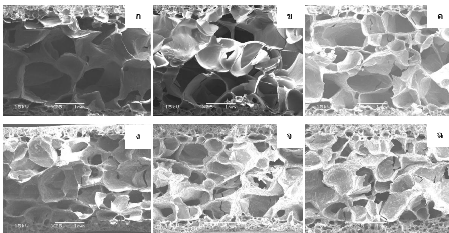
ภาพที่ 1 ภาพตัดขวางของคอมพอสิตโฟมแข็งมันสำปะหลังที่เติมผงซีลี้อย่างพหามีปริมาณต่างๆ จากกล้องจุลทรรศน์อิเล็กตรอนแบบส่องกราดที่ระดับกำลังขยาย 25 เท่า (ก) 0% (ข) 5% (ค) 10% (ง) 15% (จ) 20% และ (ฉ) 25% โดยน้ำหนักของแป้ง
