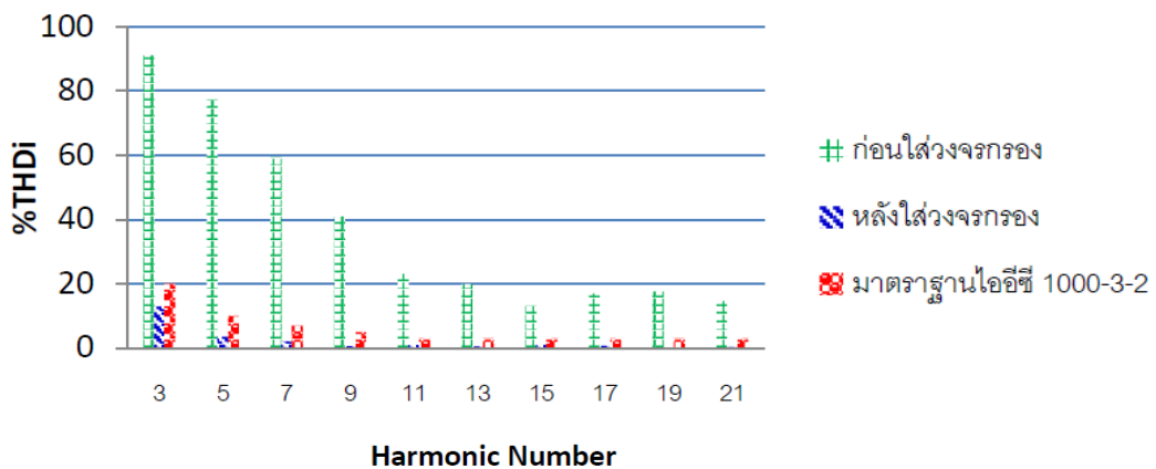
ภาพที่ 5 แสดงการเปรียบเทียบระหว่างก่อนและหลังใส่ตัวเหนี่ยวนำด้านแหล่งจ่ายกับมาตรฐาน IEC 1000-3-2
