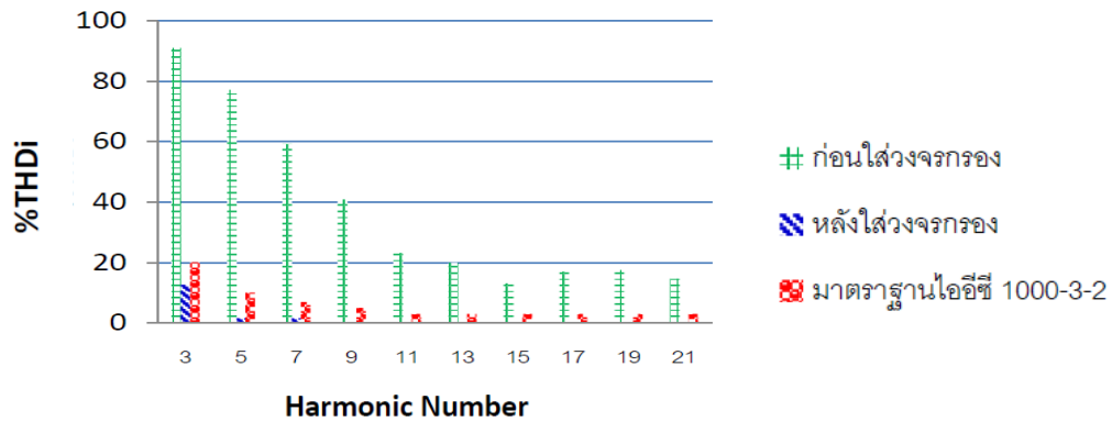
ภาพที่ 6 แสดงการเปรียบเทียบระหว่างก่อนและหลังใส่วงจรกรองแบบจูนความถี่ลำดับที่ 5 กับมาตรฐาน IEC 1000-3-2
