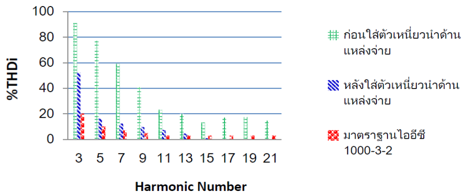
ภาพที่ 4 แสดงการเปรียบเทียบระหว่างก่อนและหลังใส่ตัวเหนี่ยวนำด้านแหล่งจ่ายกับมาตรฐาน IEC 1000-3-2
