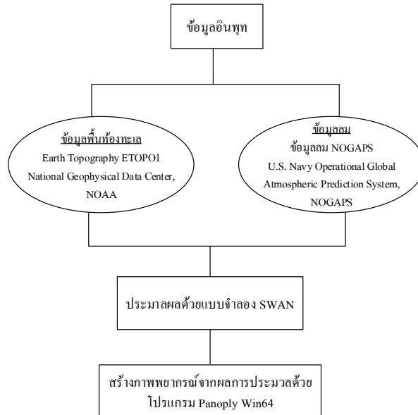
ภาพที่ 2 ไดอะแกรมแสดงการทำงานของแบบจำลองคลื่น
