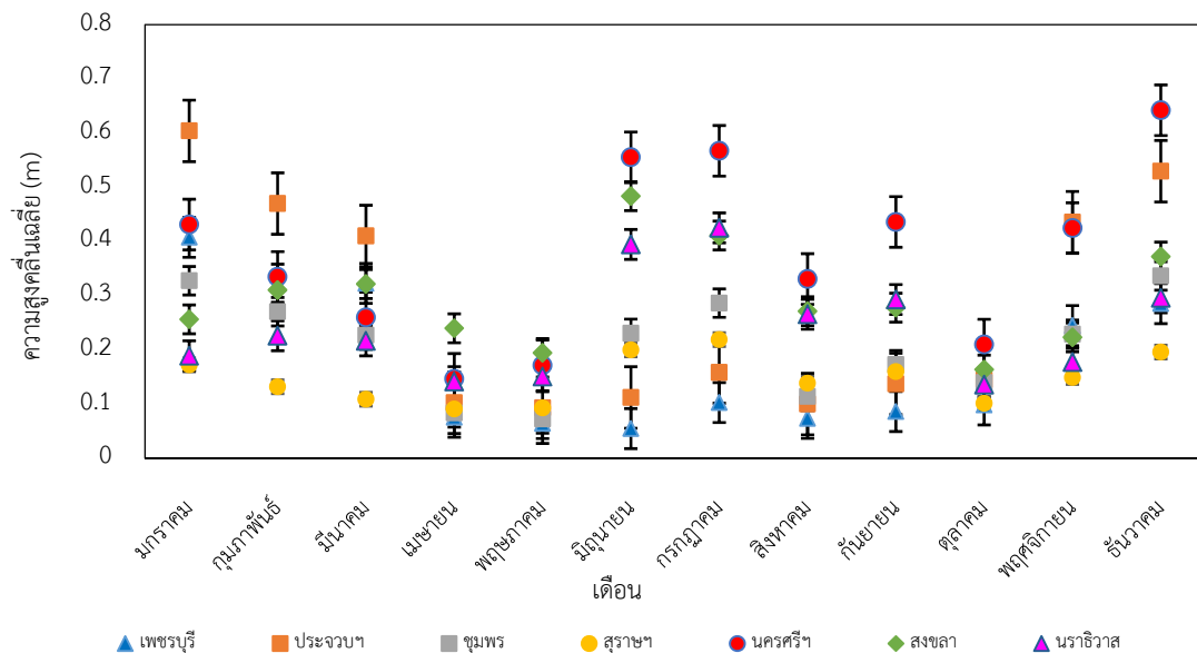
ภาพที่ 4 ค่าความสูงคลื่นนัยสำคัญเฉลี่ยรายเดือน ปี ค.ศ.2014
