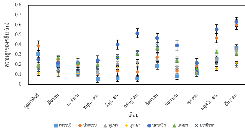
ภาพที่ 3 ค่าความสูงคลื่นนัยสำคัญเฉลี่ยรายเดือน ปี ค.ศ.2013
