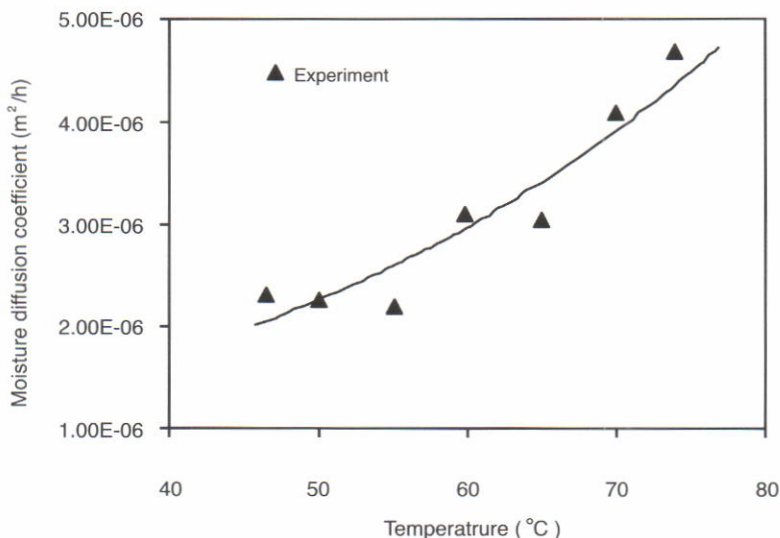
รูปที่ 4 แสดงค่าสัมประสิทธิ์การแพร่ความชื้นที่อุณหภูมิต่างๆ จากผลการทดลองที่ความเร็วลม 1.3 m/s และจากสมการแบบจำลองสัมประสิทธิ์การแพร่ความชื้นของจิง
