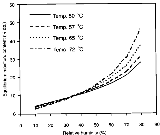
รูปที่ 1 แสดงลักษณะเส้นความชื้นสมดุลไอโซเทอมของจึงด้วยรูปสมการของ Oswin , 1946 [20]
