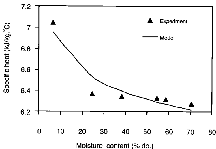
รูปที่ 3 แสดงการเปรียบเทียบระหว่างผลการทดลองและแบบจำลองความร้อนจำเพาะของขิงที่ความชื้นต่างๆ
