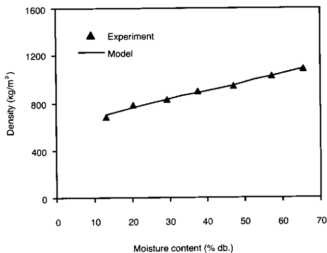
รูปที่ 2 แสดงการเปรียบเทียบระหว่างผลการทดลองและแบบจำลองความหนาแน่นของจึงที่ความชื้นต่างๆ
