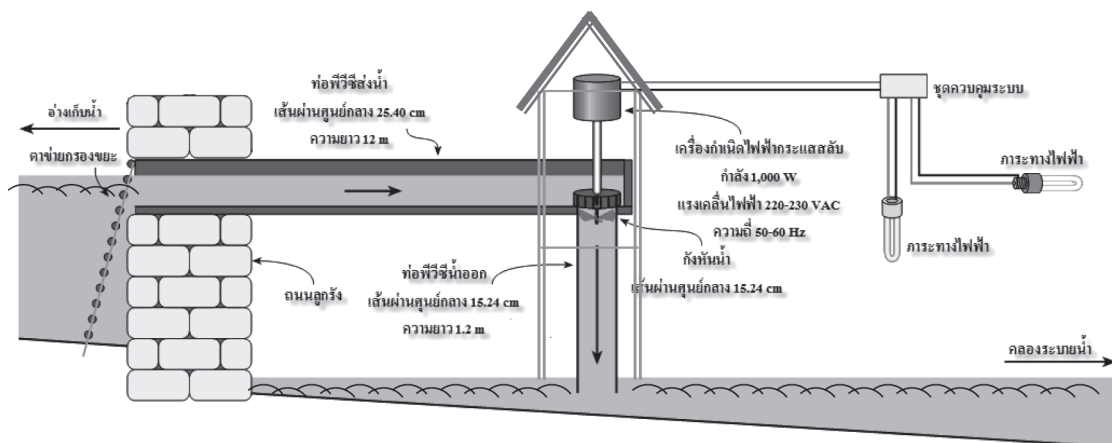
รูปที่ 3 ภาพจำลองระบบผลิตไฟฟ้าพลังงานน้ำขนาดเล็ก ณ มูลนิธิ สุข-แก้ว แก้วแดง
